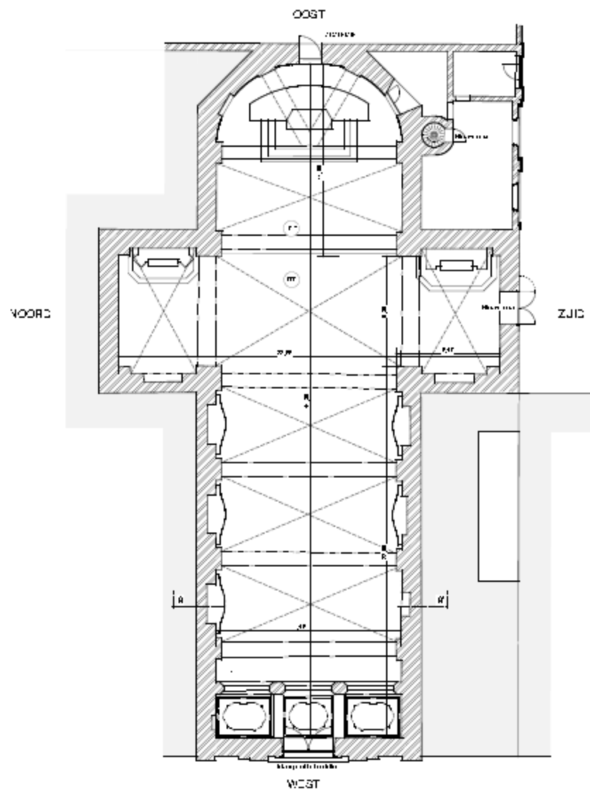
GRONDPLAN
